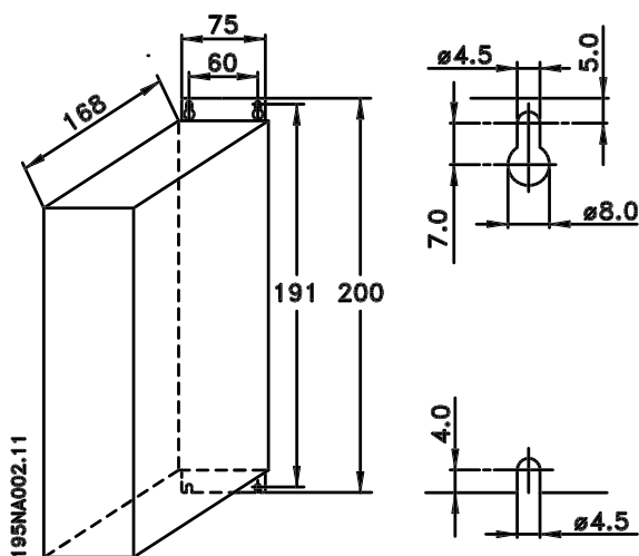
VLT 2805-2815 380-480V
